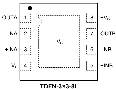
UDL6518D (TOP VIEW)
