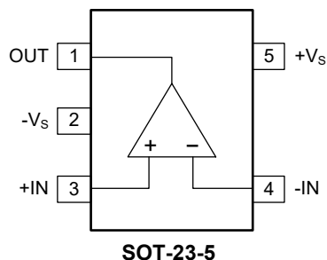
UDL6518 (TOP VIEW)
