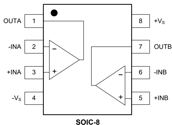
UDL6518D (TOP VIEW)
