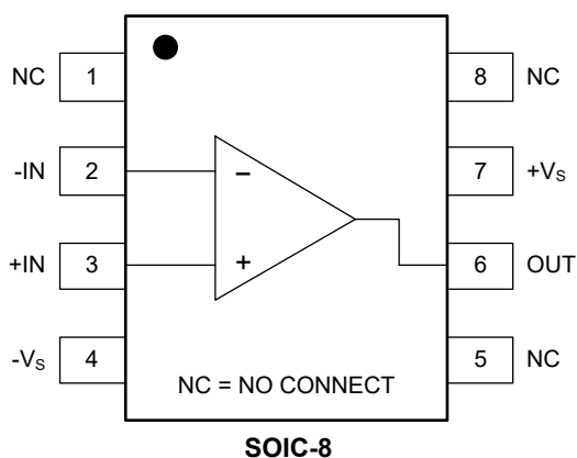
UDL6518 (TOP VIEW)
