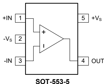
UDL6518 (TOP VIEW)
