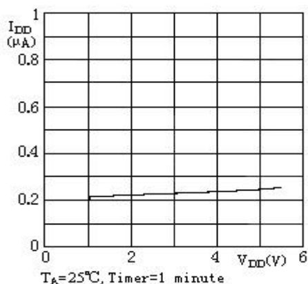
CLKOUT禁止时, I_{DD} 与 V_{DD} 的关系图
