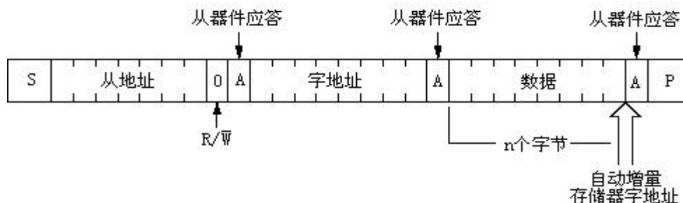
图15. 主发送器到从接收器（写模式）
