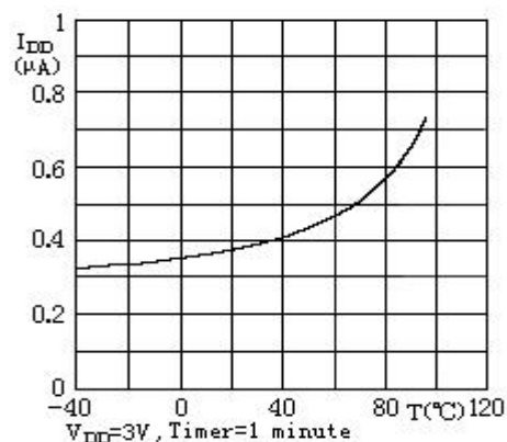
CLKOUT=32.768kHz, I_{DD} 与 T_A 关系图
