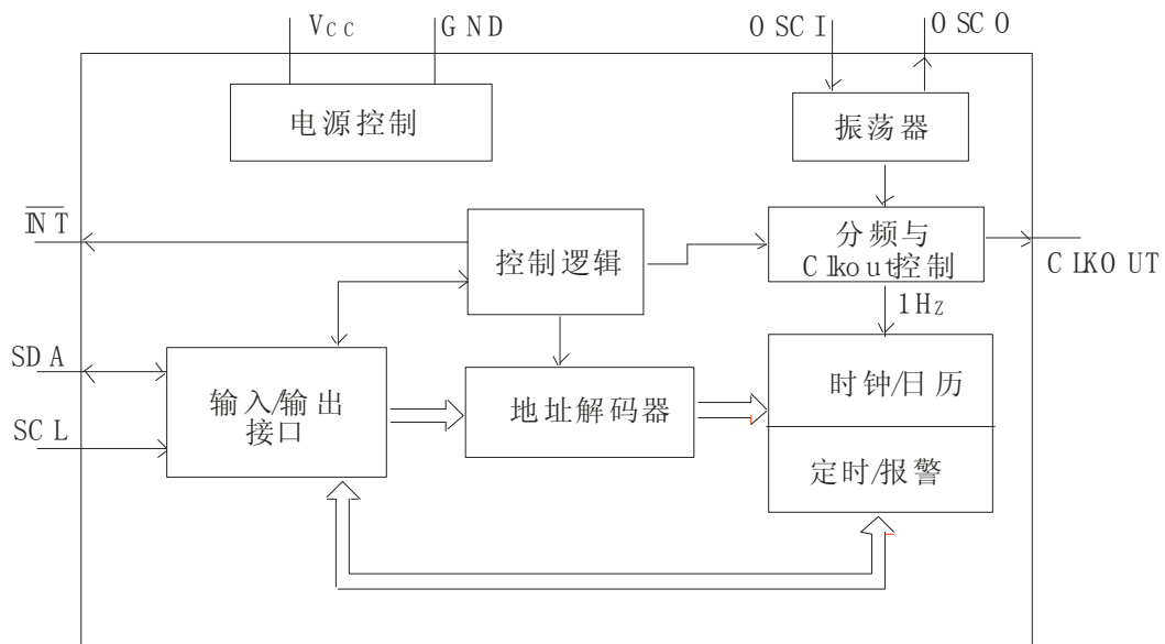
图 2. 方框图
