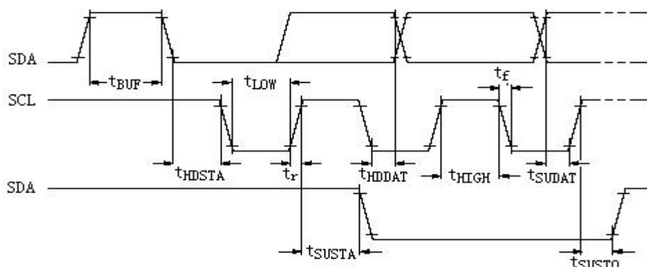
图 4 I 2 C 总线时序波形
