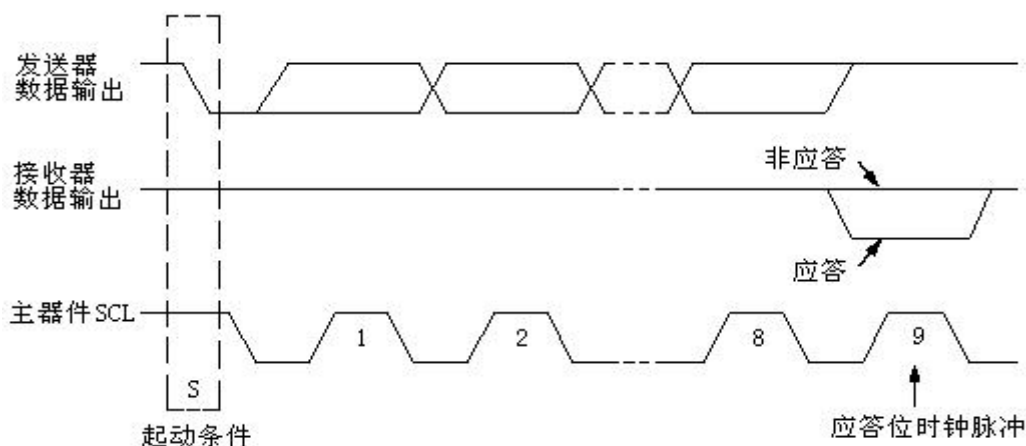
图13. I2C总线的应答位
