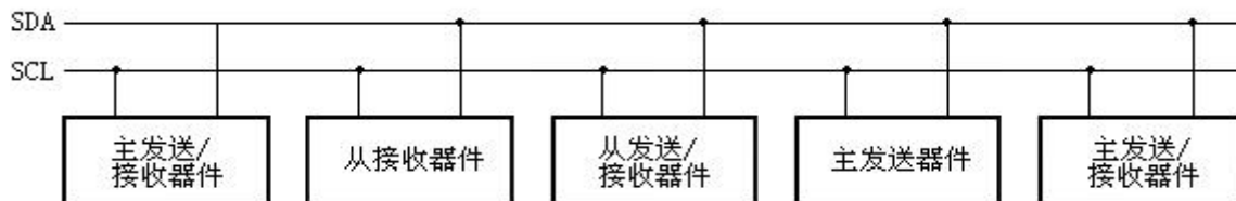
图10. I2C总线系统配置图
