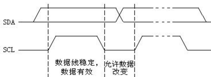
图12. I2C总线上的位传送
