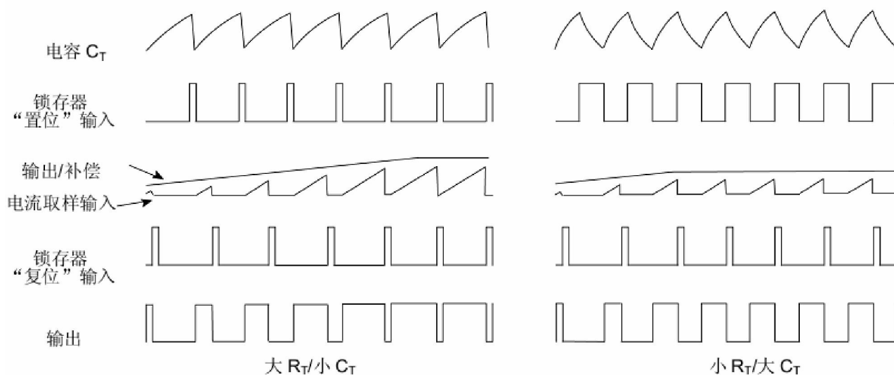
图 18. 时序图
